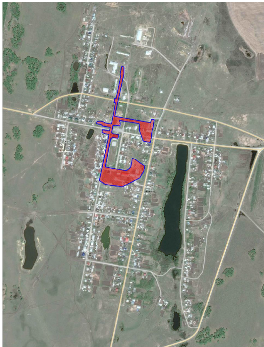
Рисунок 1.1 – Существующие и перспективные зоны действия источников теплоснабжения на территории поселка Новый Урал
