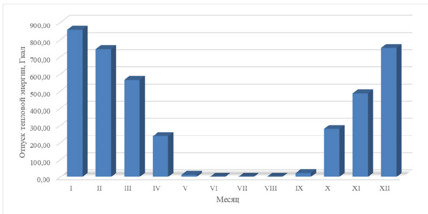
Рисунок 1.3 – Оптимальный график помесячного отпуска тепловой энергии для Котельной «Новый Урал»
